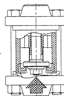
垂直 (入口下側)
