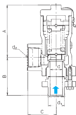
25A 突合せ溶接
