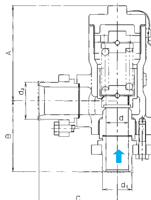
32A~65A 突合せ溶接
