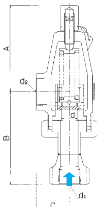
10A~20A 10A-H~15A-H ねじ込み型
