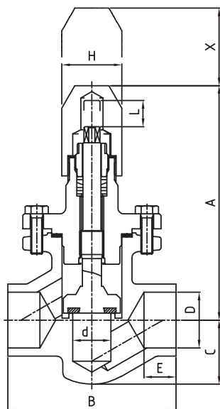
10A~25A 差込み溶接
