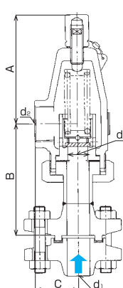
10A~20A RTKフランジ型
